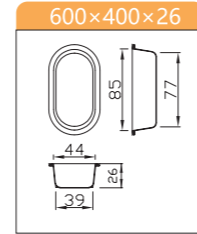
SN9089 ¥11,210 36連楕円型 アルタイト シリコン 600x400x26 中型 85x44x26
